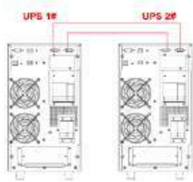
Şekil 2-3: 2 UPS Paralelli Sistem
