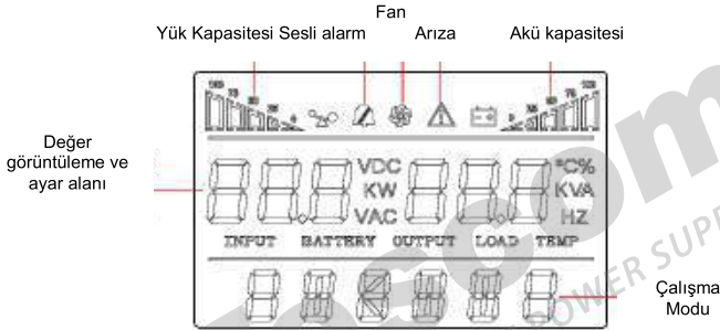
Şek. 3- 2: LCD Menüsü
