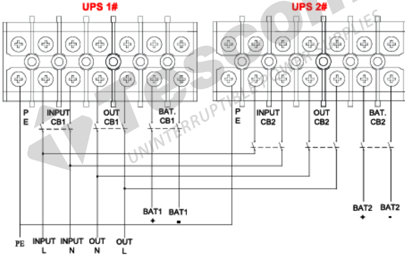
Şek. 2- 2: Paralel Kablolama Şeması
