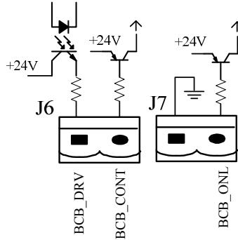
Şekil 3-21 BCB Portu
