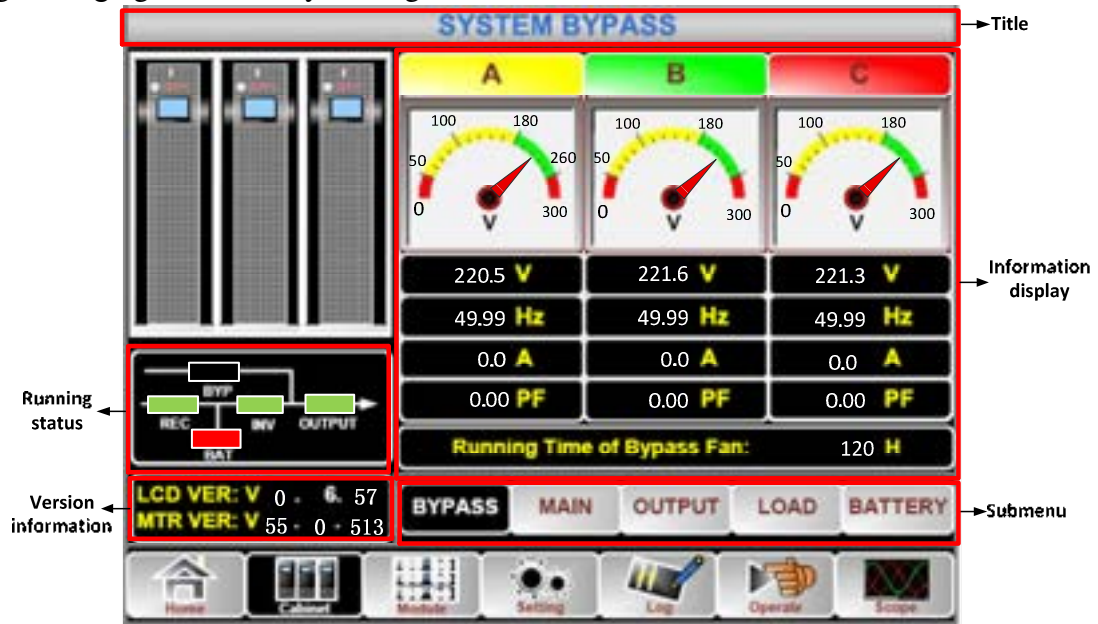
Şekil 4-6 Kabin
