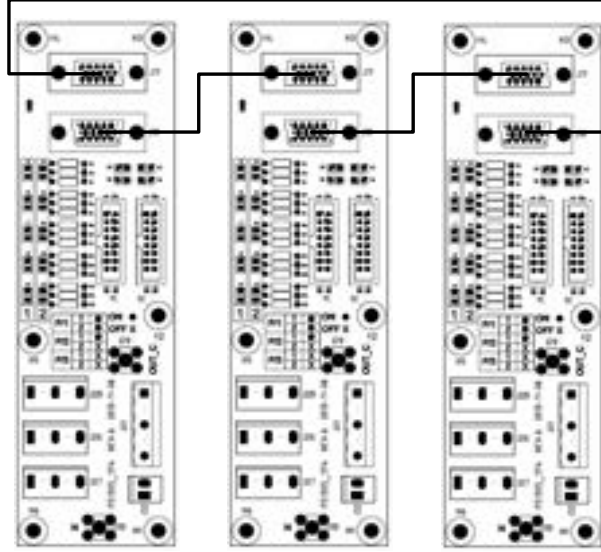
Şekil 5- Paralel bağlantı
