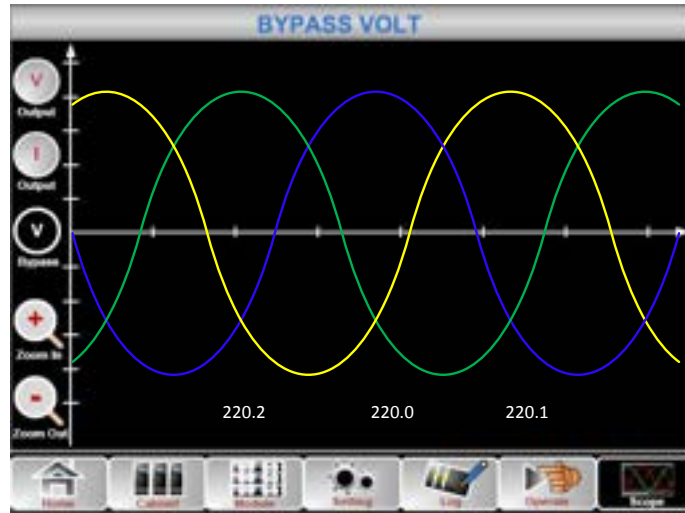
Şekil 4-13 Osiloskop Menüsü
