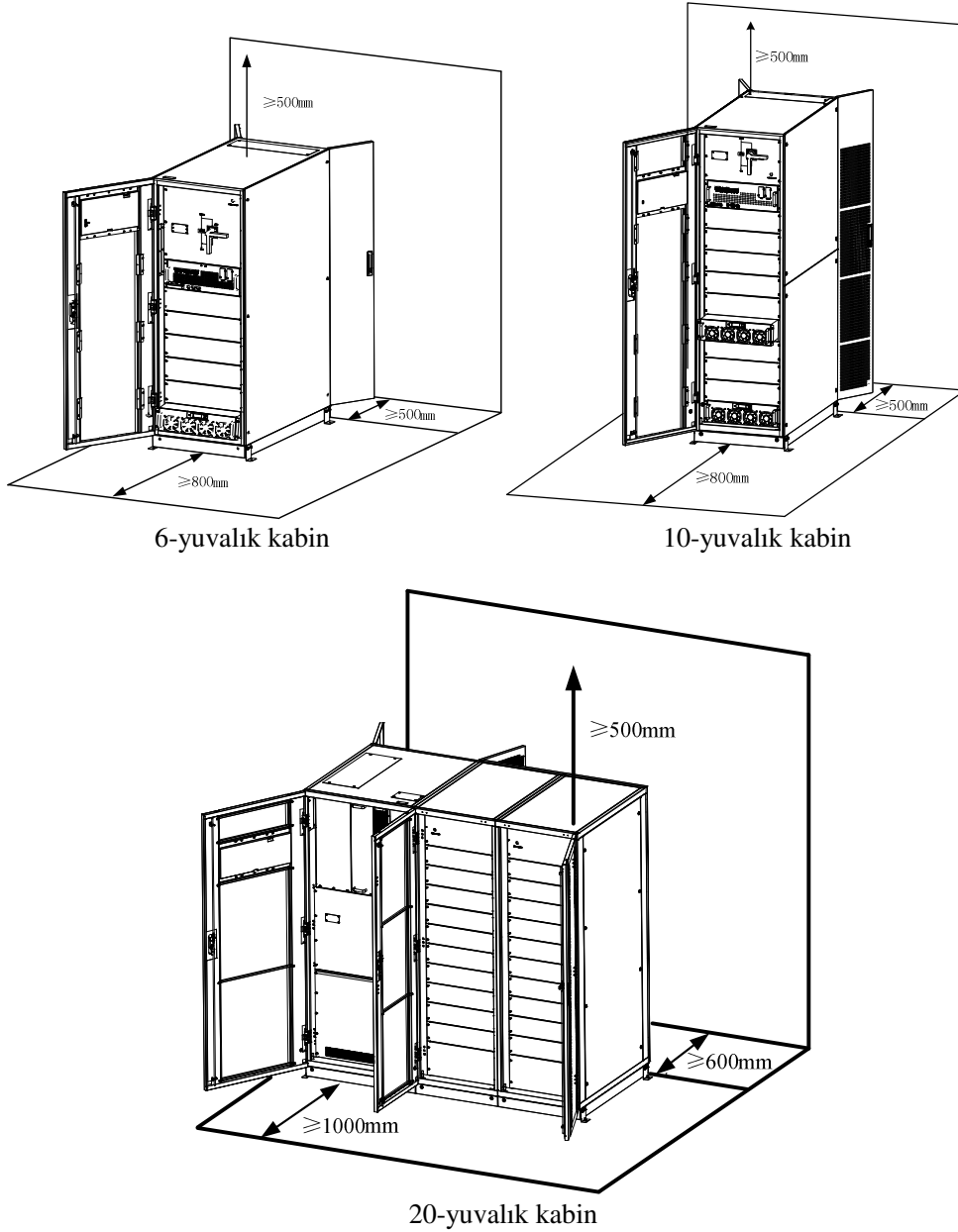
Şekil3-1 Kabin için ayrılan alan (Birim: mm)
